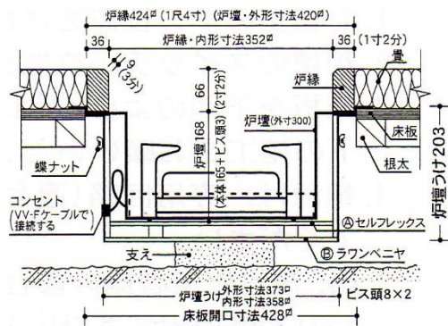
炉壇受け16型施工図 ※詳しい施工方法は製品に同封されております
