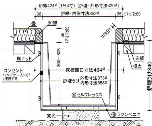
炉壇受け30型施工図 ※詳しい施工方法は製品に同封されております
